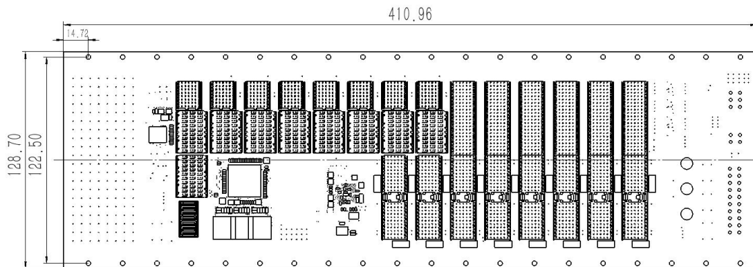
图 10 机箱 14 槽背板效果图
