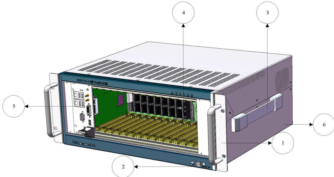
图1 RX39114 外观图
