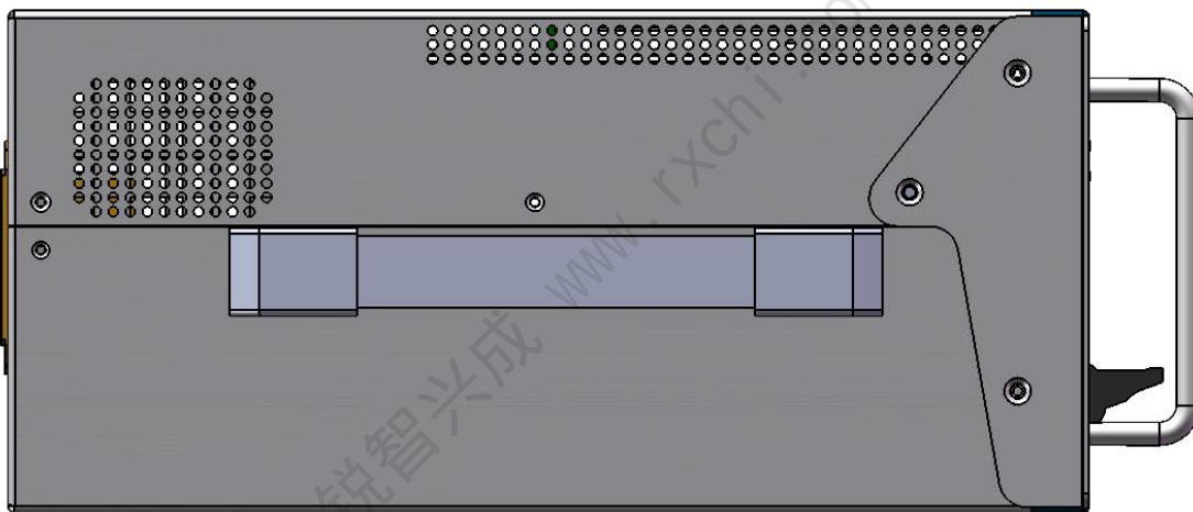
图 8 机箱侧视图
