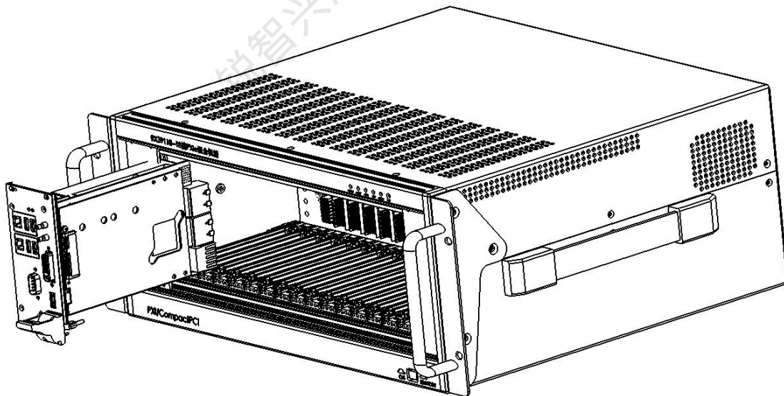
图 9 控制器安装示意图
